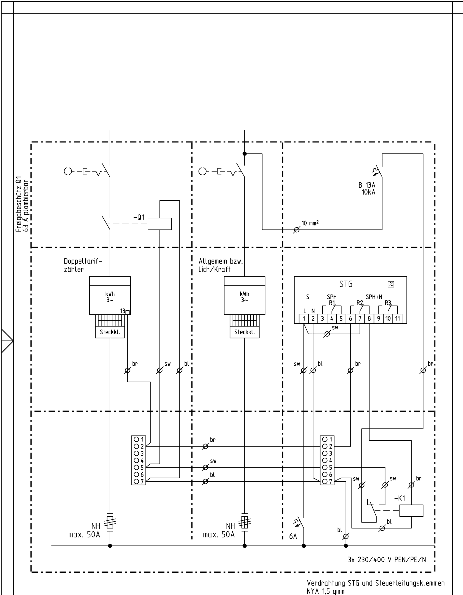
Verdrahtungsplan allgemeine steuerbare Verbrauchereinrichtung gemäss § 14a EnWG
